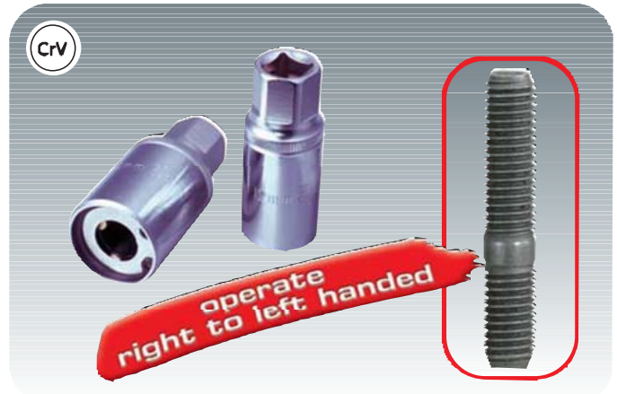
1/2" Stud puller
